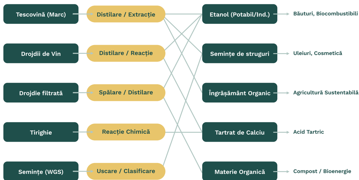
Diagrama Fluxului Tehnologic Bioaldevin
